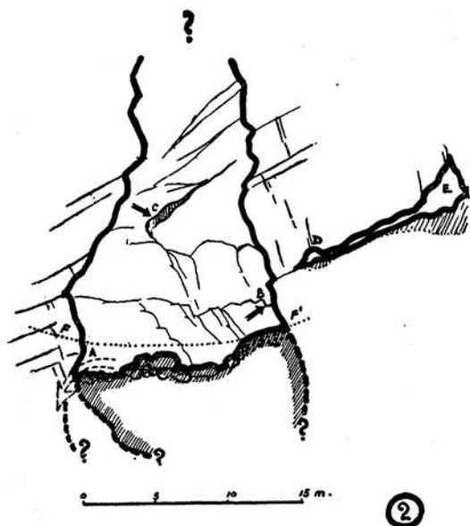
Figura 6.—CORTE I-I'
